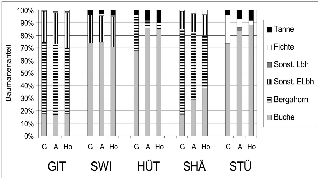
Abb. 3: Baumartenanteile in der Verjüngung nach Schichtung; G: Gesamtpflanzen, A: A-Schicht mit Pflanzen, deren Höhen mindestens 80 % der Höhe der höchsten Pflanze (Maximalhöhe) je Kleinfläche erreichen (=herrschende Verjüngungsschicht), Ho: jeweils höchste Pflanze pro Kleinfläche
