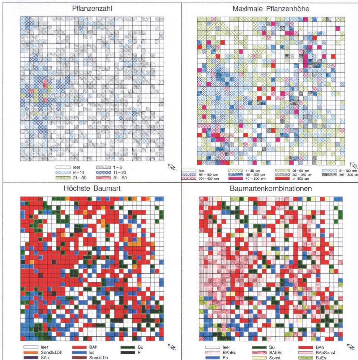
Abb. 4: Verjüngung in der Repräsentationsfläche des NWRes Gitschger; Aufnahme­fläche 80 m x 80 m; 1024 Klein­flächen je 2.5 m x 2.5 m
